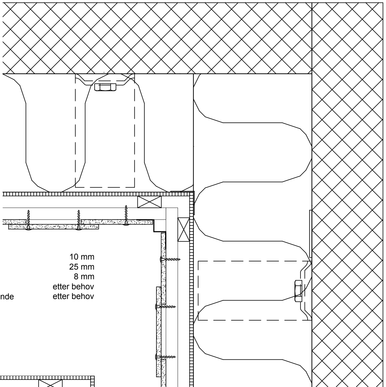
konstruksjonsprinsipp 1 med hjørneprofil.
