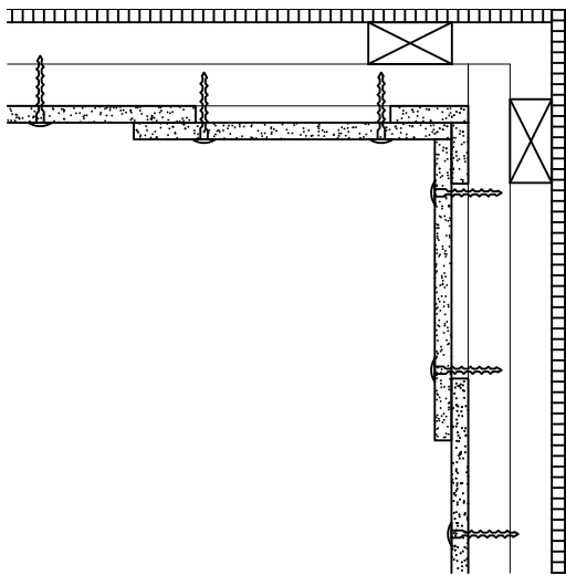
Konstruksjonsprinsipp 2 uten profiler.
